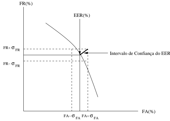
FIG. 5.5: Intervalo de confiança do EER.
